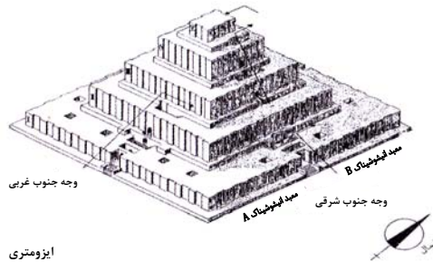
نما، پرسپکتیو و پلان زیگورات چغازنبیل
